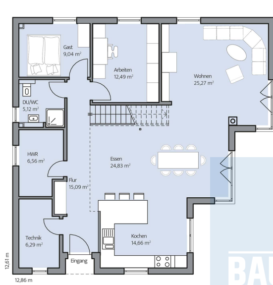
Haus Nelsen Grundriss
